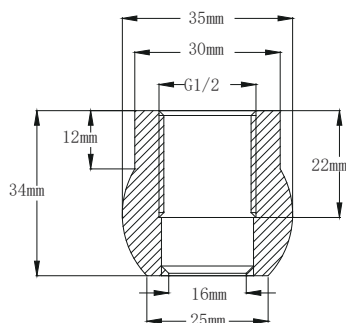
焊接底座
