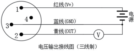
电压输出接线图（三线制）
