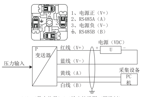
RS485（数字信号）8-6输出接线图（四线制）
